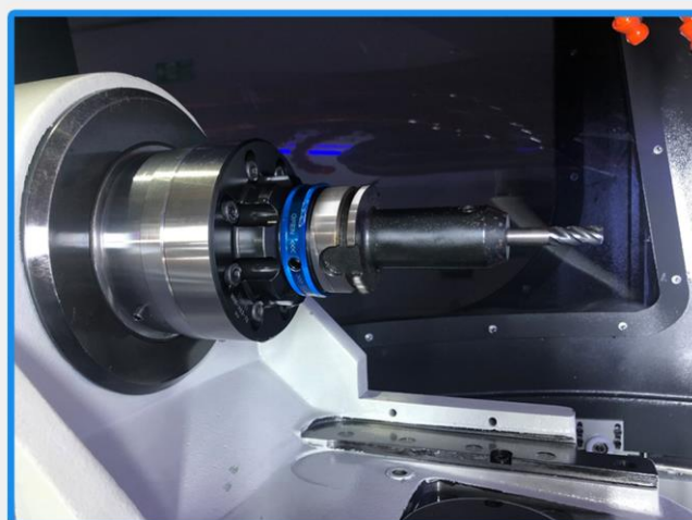
HSK - A63 Держатель инструмента
