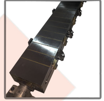
Manyetik Tabla Üzerinde T-Slotlu Mekanik Bağlantı Sistemi
