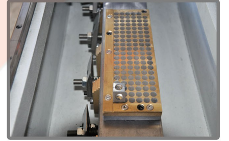
Takma Uçlar İçin Opsiyonel Manyetik Aparatı
