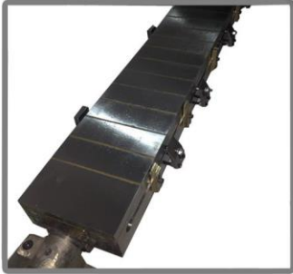
Manyetik Tabla Üzerinde T-Slotlu Mekanik Bağlantı Sistemi
