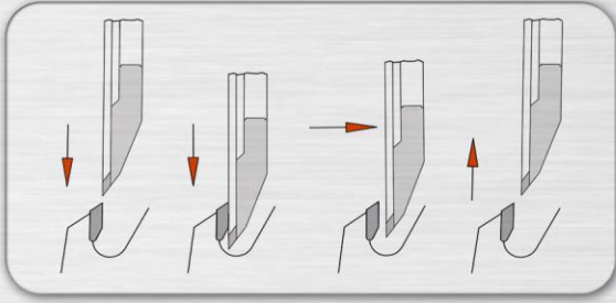
İç Bileme
