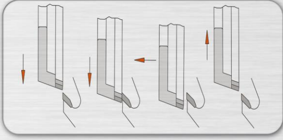
Sırt Bileme
