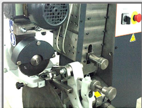
Chanfragem manual direita/esquerda de serras circulares HSS
