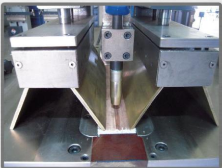
Controlled annealing process during welding on the same welding table Proceso de recocido controlado durante la soldadura en la misma mesa Processo de revenido controlado durante a solda na mesma mesa
