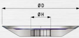
İç bileme taşı Tip: 12V2 D: Ø 100-125 mm d: Ø 20 mm
